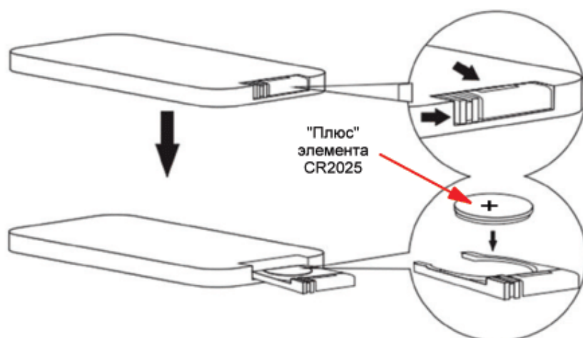
Рис.2. Установка элемента питания.
