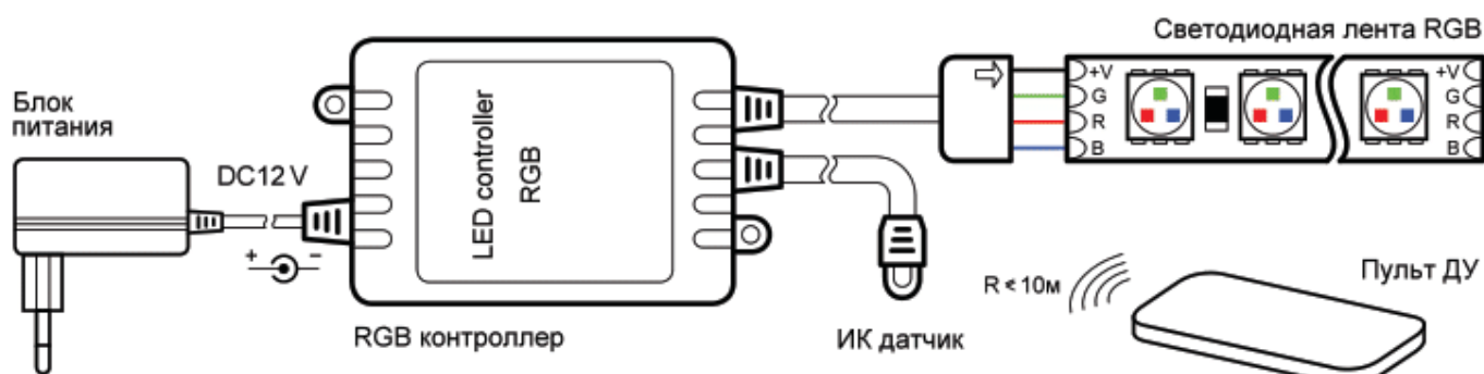
Рис.1. Схема подключения.
